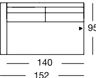
ASO 170/152
